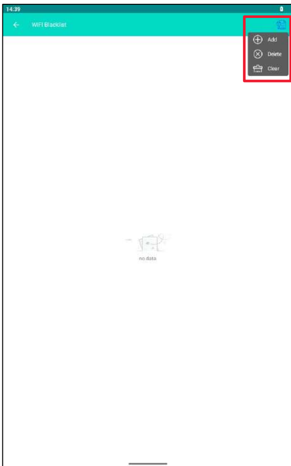
Рисунок 90. WIFI Blacklist
