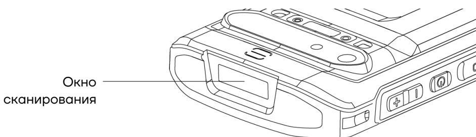
Рисунок 171. Окно сканирования
