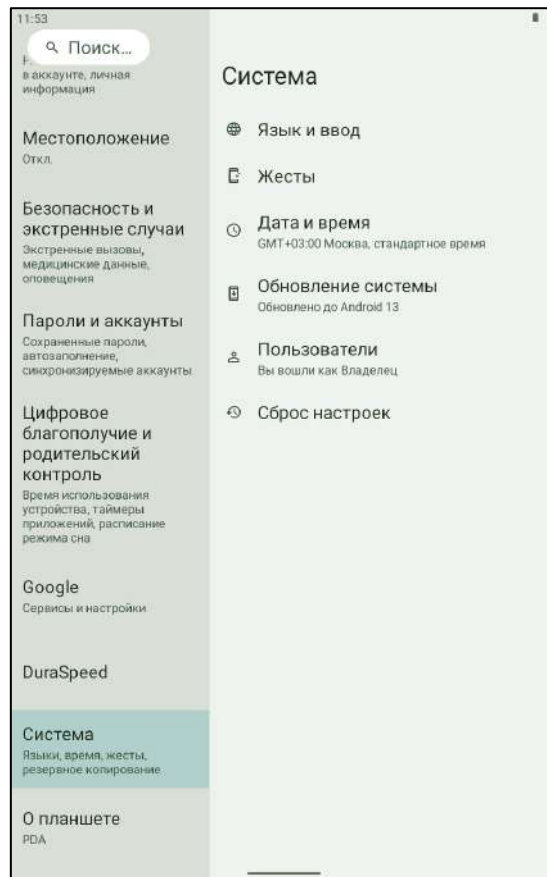
Рисунок 47. Система
