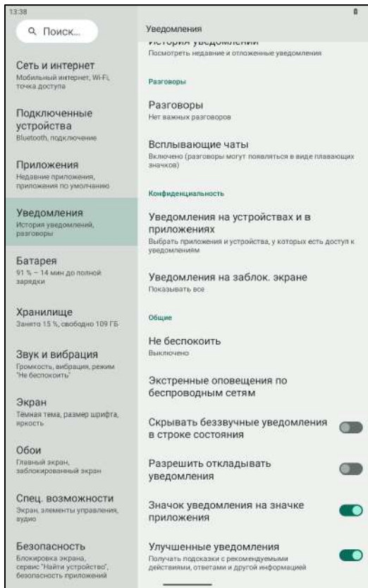
Рисунок 27. Уведомления. Продолжение
