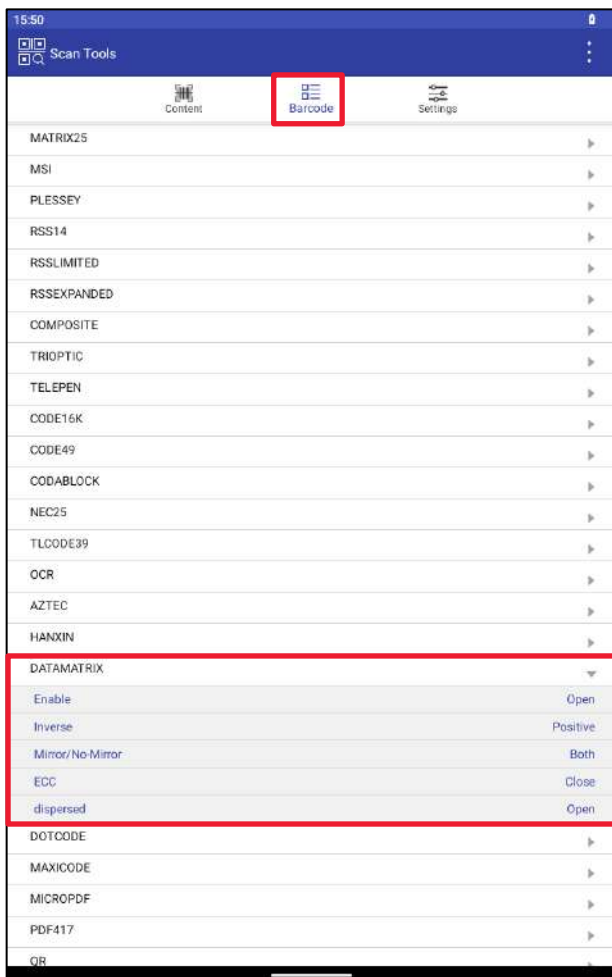
Рисунок 165. DATAMATRIX
