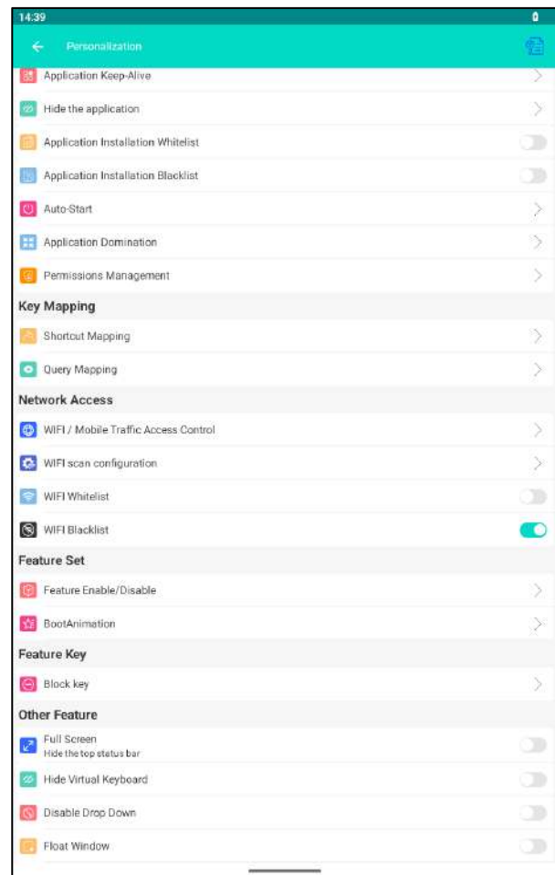
Рисунок 91. WIFI Blacklist
