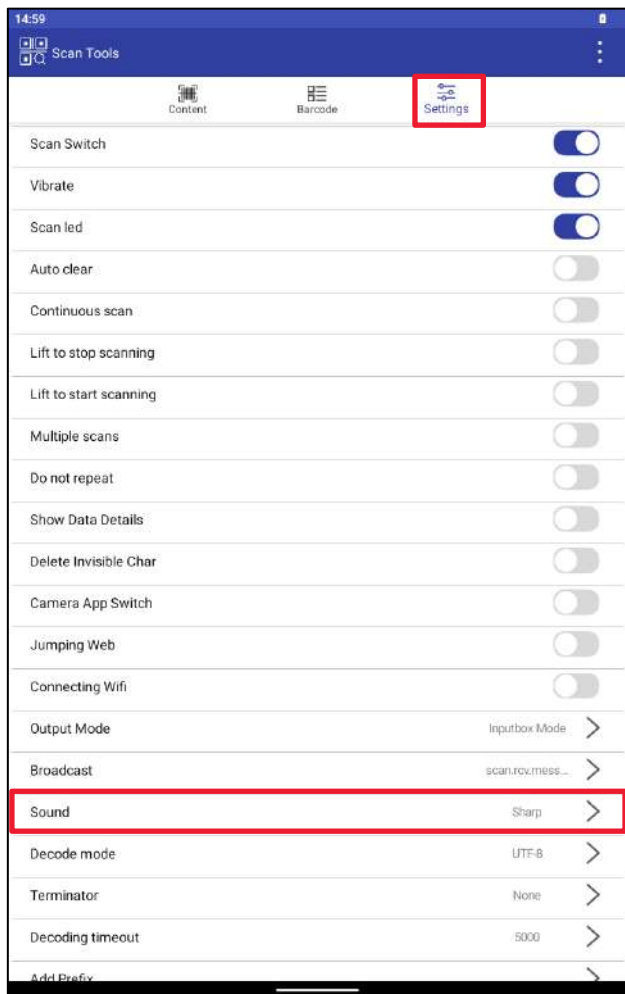
Рисунок 119. Settings. Sound
