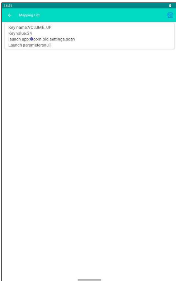
Рисунок 83. Query mapping
