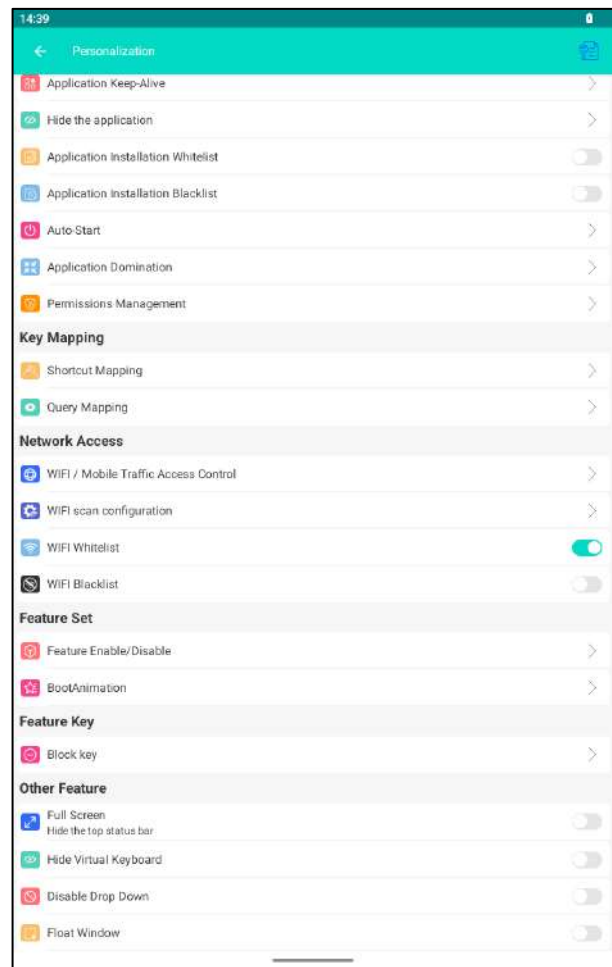
Рисунок 89. WIFI Whitelist
