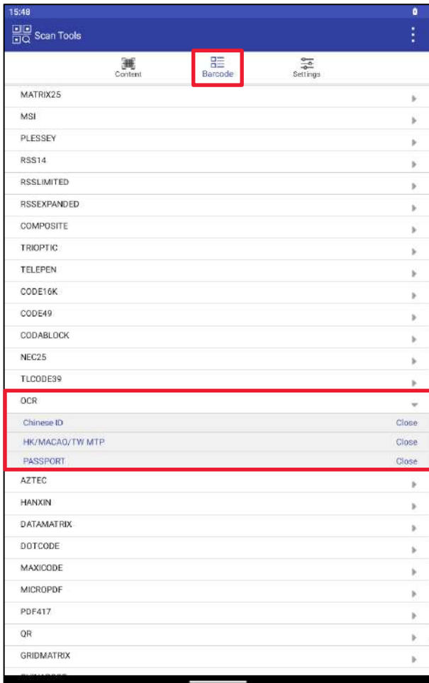
Рисунок 163. OCR
