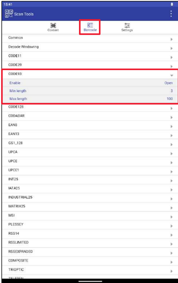
Рисунок 144. CODE93
