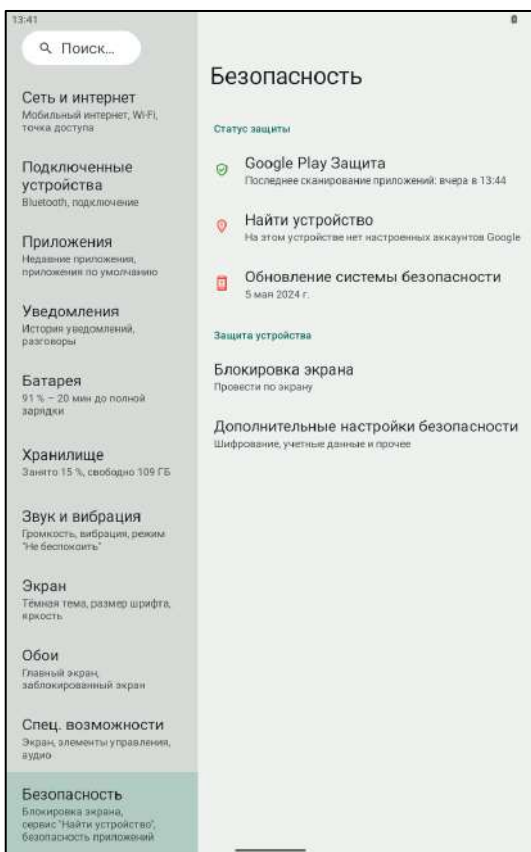
Рисунок 37. Безопасность
