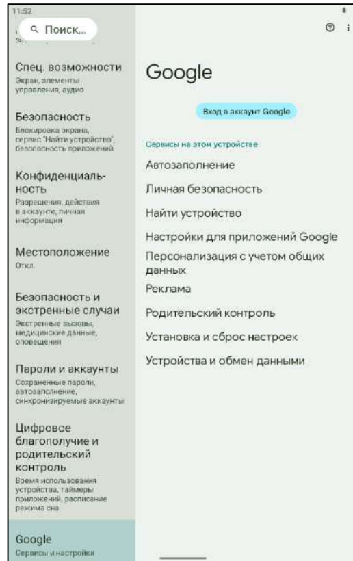
Рисунок 45. Google
