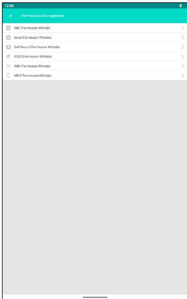
Рисунок 68. Permission Management
