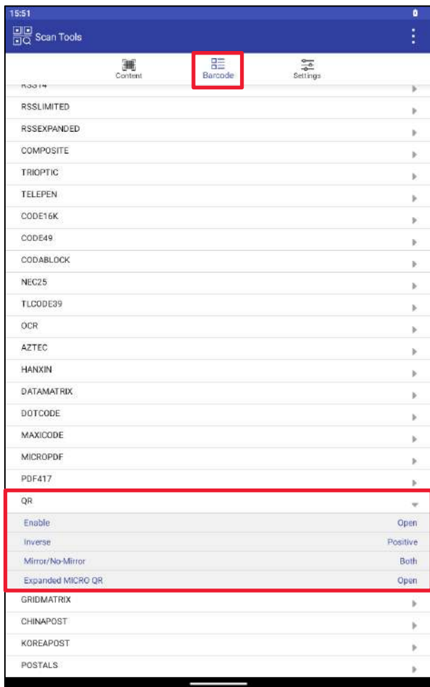
Рисунок 166. QR
