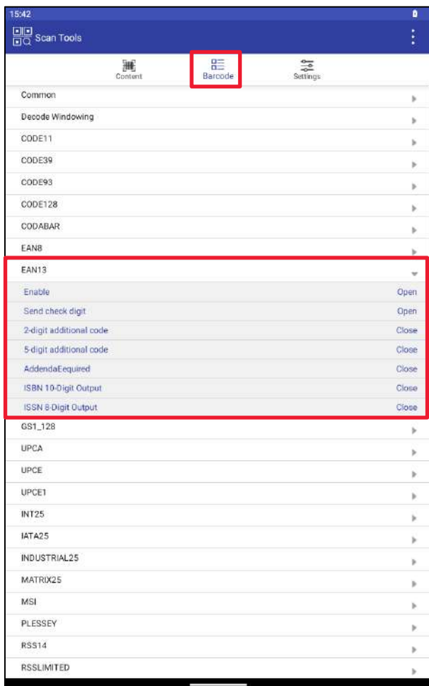
Рисунок 148. EAN13
