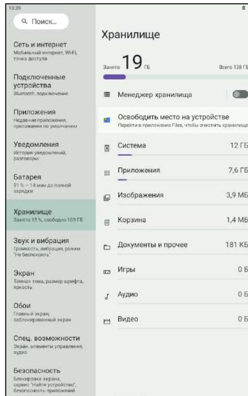
Рисунок 30. Хранилище
