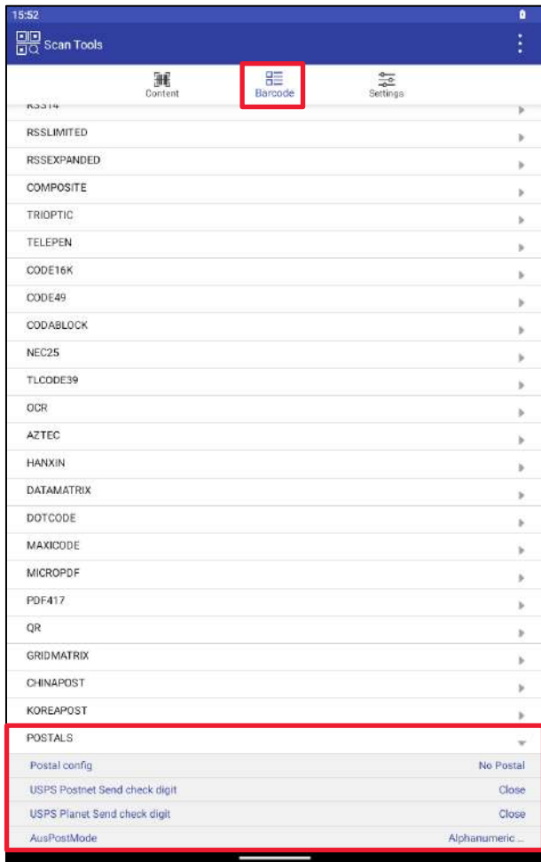
Рисунок 170. POSTALS
