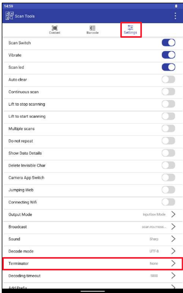
Рисунок 121. Settings. Terminator
