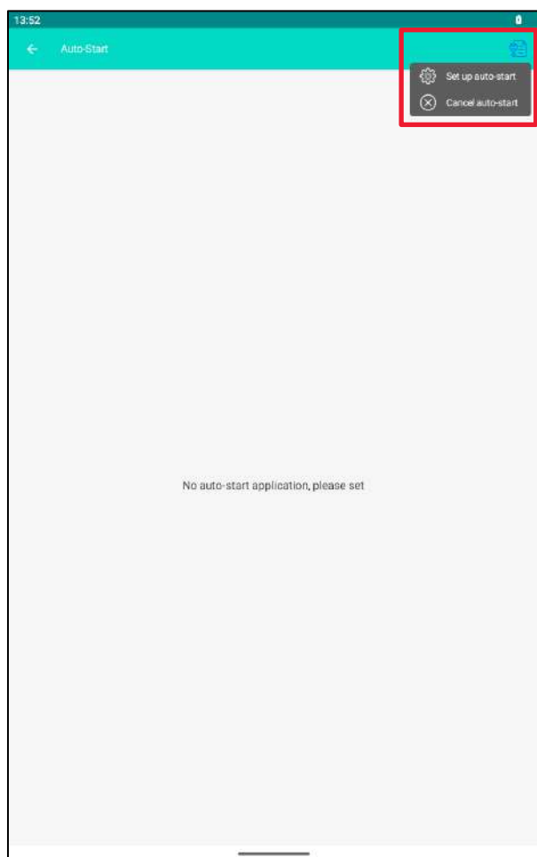
Рисунок 64. Auto-Start
