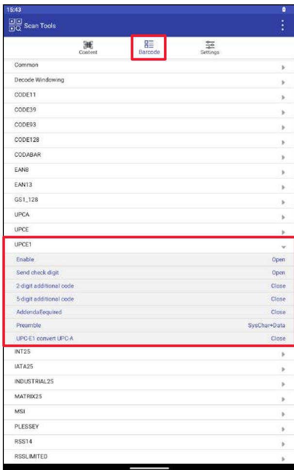
Рисунок 152. UPCE-1
