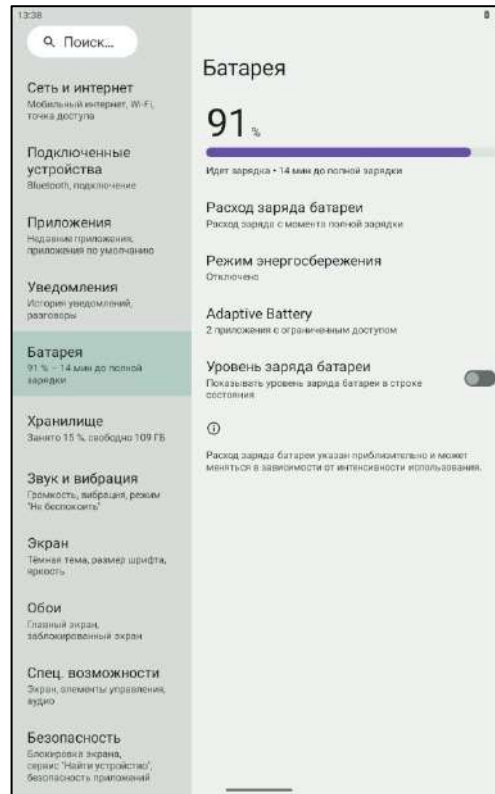
Рисунок 29. Батарея
