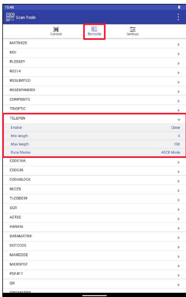
Рисунок 161. TELEPEN
