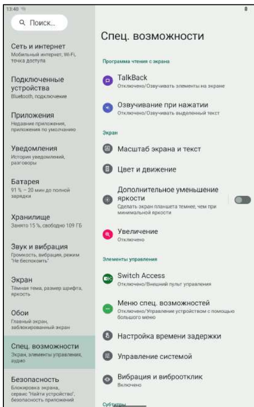
Рисунок 35. Спец. возможности
