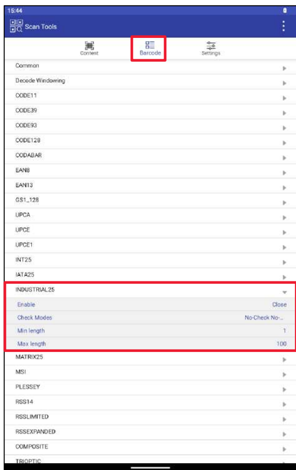
Рисунок 155. INDUSTRIAL25
