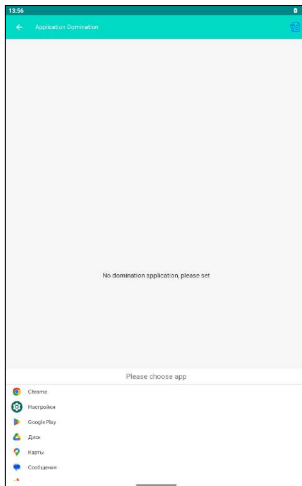
Рисунок 67. Application Domination
