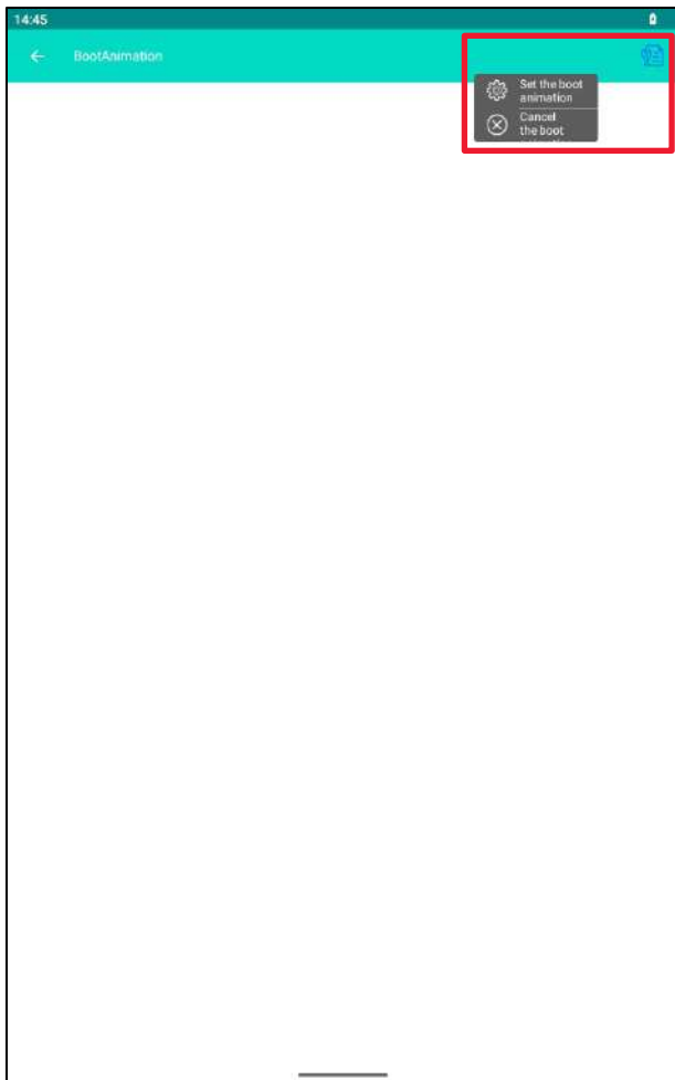
Рисунок 93. BootAnimation
